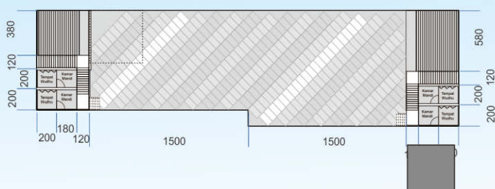
Lantai Bawah
